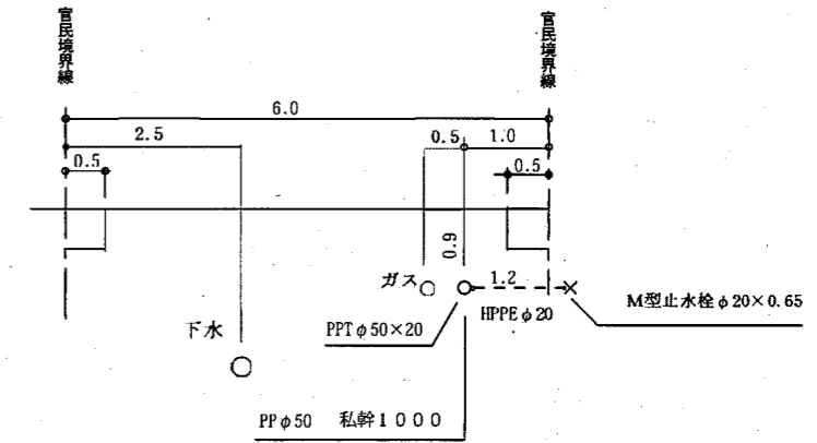
横断面図 1:100
