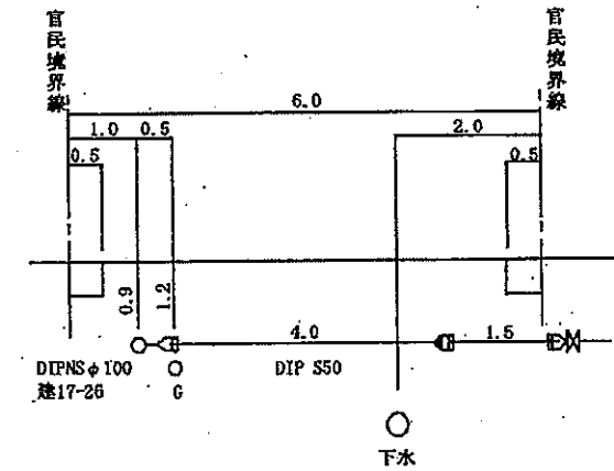
横断面図 1:100
