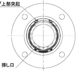
ロックリングの突起位置
