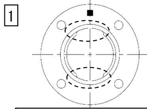
ロックリングの突起位置
