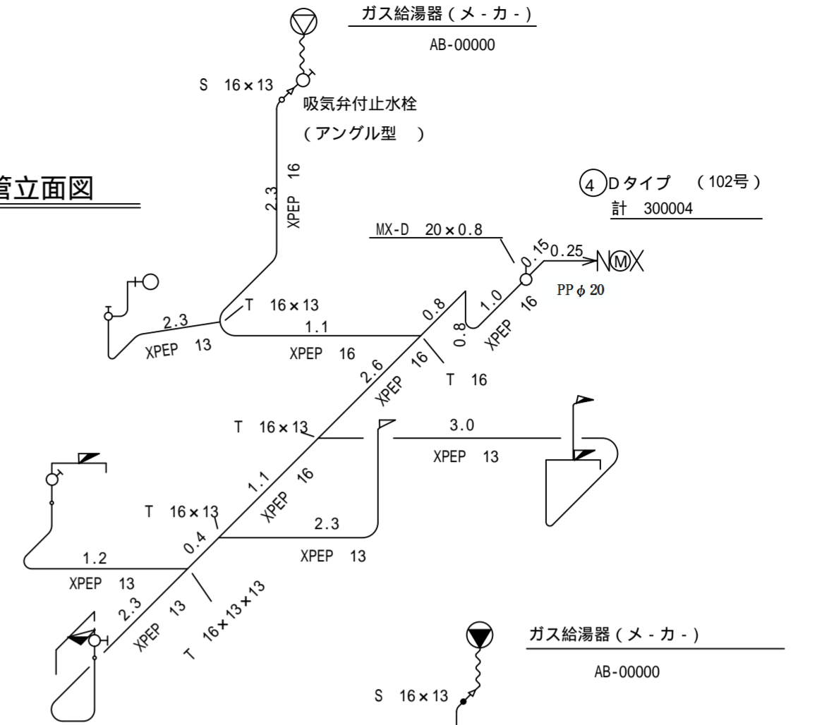
Dタイプ 平面図
