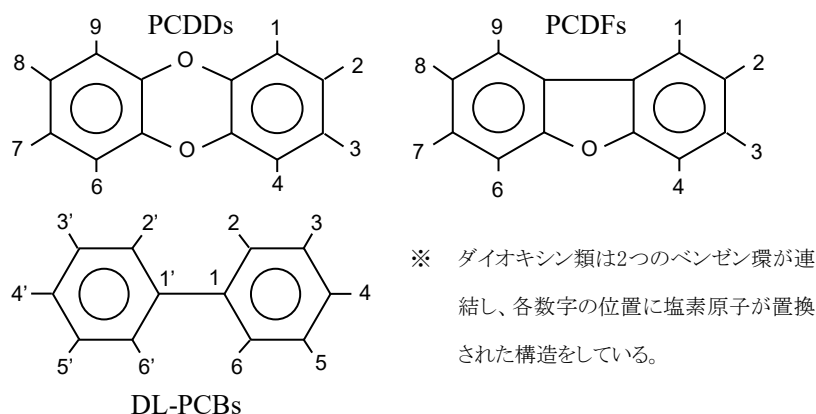
図2-6-1 ダイオキシン類の一般的な分子構造
