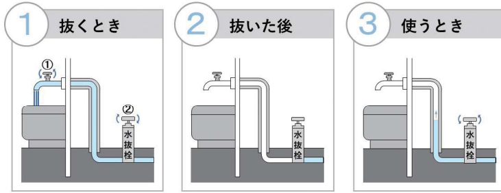
①蛇口をいっぱいに開け水を出す ②水抜栓のハンドルを時計回りに止まるまで回す ③蛇口を開けたままにしておく 水抜栓のハンドルを反時計回りに止まるまで回す
