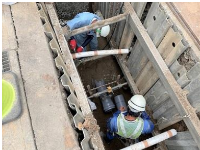
汚水管布設工事
