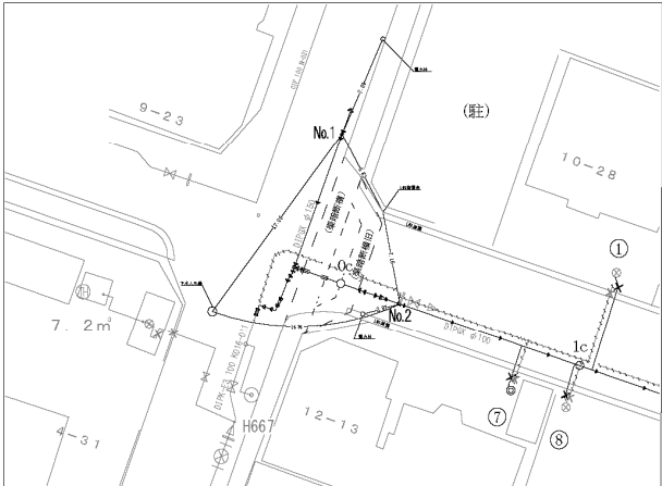
仕切弁No.1～2
